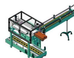
AEB-III Automatic Carton Filler 自动装箱机 (散落式装箱) Speed/封箱速度: 5 \sim 10\text{箱/分}
